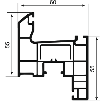
Yağ 006 Kanat Profili / Sash Profile
