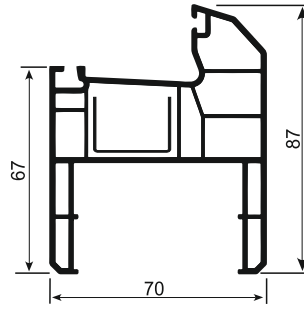
Yağ 012 U Kasa Profili / U Frame Profile
