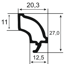
D 011 20 mm Dekoratif Çift Cam Çıtası / 20 mm Decorative Double Glazing Bead
