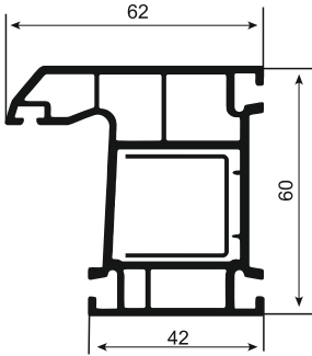
Yağ 001 Kasa Profili / Frame Profile
