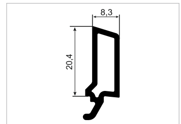
S011 24 mm Çift Cam Çıtası 24 mm Double Glazing Bead
