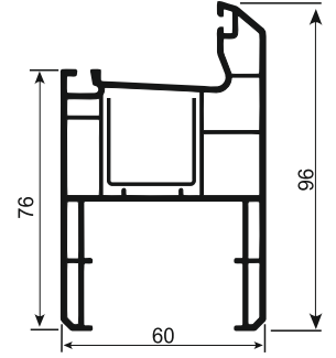
Yağ 013 U Kasa Profili / U Frame Profile
