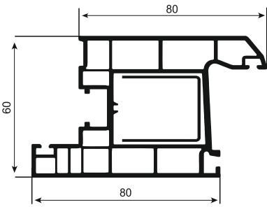
Yağ 004 Kilitli Kapı Profili / Door Sash Profile
