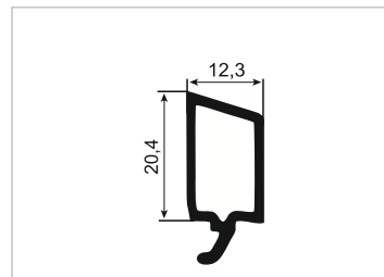
S010 20 mm Çift Cam Çıtası 20 mm Double Glazing Bead
