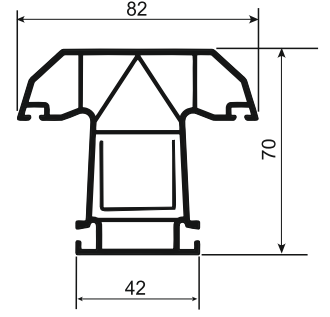
Yağ 011 Orta Kayıt Profili / Mullion Profile
