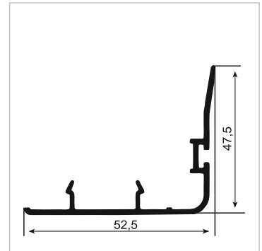
S008 Sürme Kanat Adaptörü Sliding Sash Adaptor
