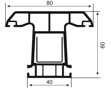
Yağ 003 Orta Kayıt Profili / Mullion Profile
