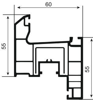
Yağ 005 Kanat Profili / Sash Profile
