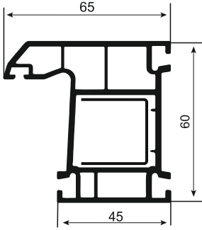
Yağ 009 Geniş Kasa Profili / Wide Frame Profile
